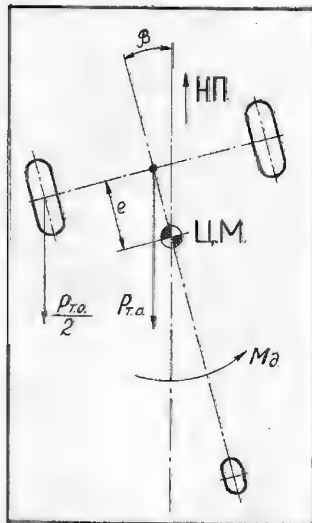
Рис.3. Схема образования destabilизирующего момента M_d (хвост поднят).
